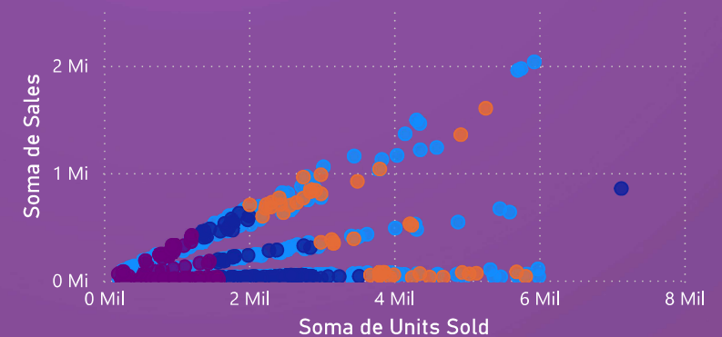
Soma de Units Sold e Soma de Sales por Profit e Profit (clusters)
